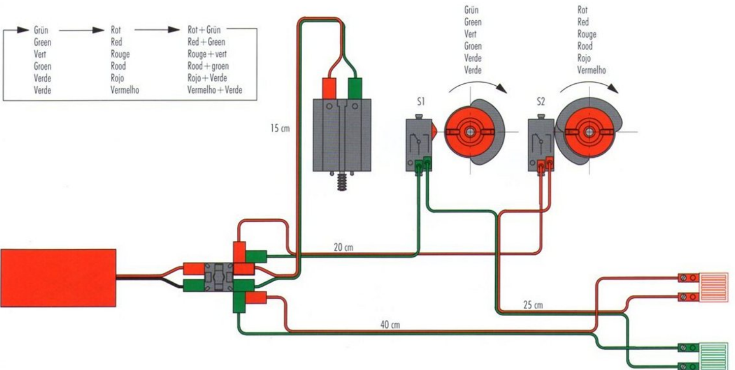
Schaltplan Circuit diagram Plan électrique
